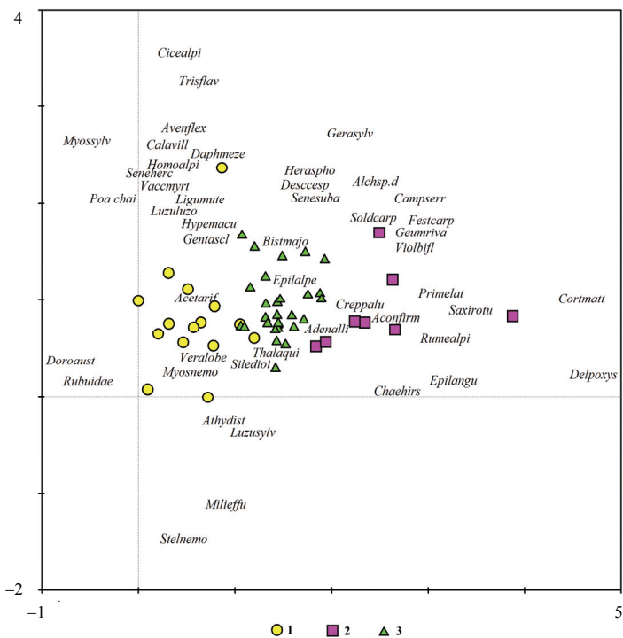
Obr. 2. Ordinačný graf nepriamej gradientovej analýzy (DCA) 51 zápisov z asociácie Aconito firmi-Adenostyletum z územia Krivánskej Fatry. Eigenvalues: 1. os 0,441, 2. os 0,199, dĺžka gradientu: 1. os 3,875, 2. os 2,368. Zobrazené sú druhy s váhou > 1 %. 1 – variant s Doronicum austriacum , 2 – variant s Delphinium oxysepalum , 3 – typický variant
